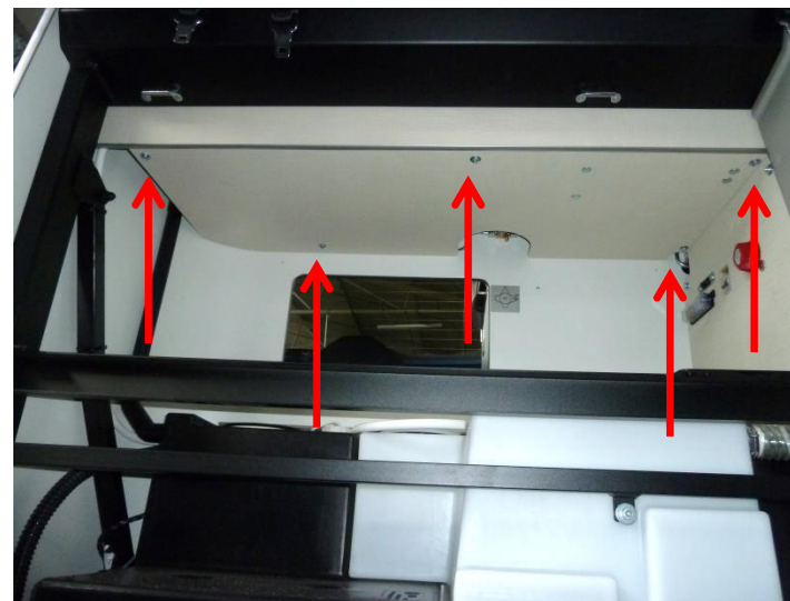
5 Schrauben entfernen
