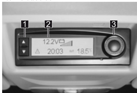
Abb.: Zentralelektronik
