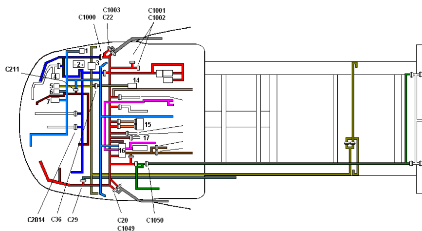
Bild 2: Pritschenwagen, Benzinmotor
