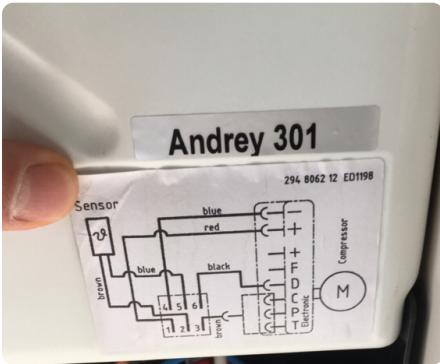
Der Schaltplan des Kühlschranks
