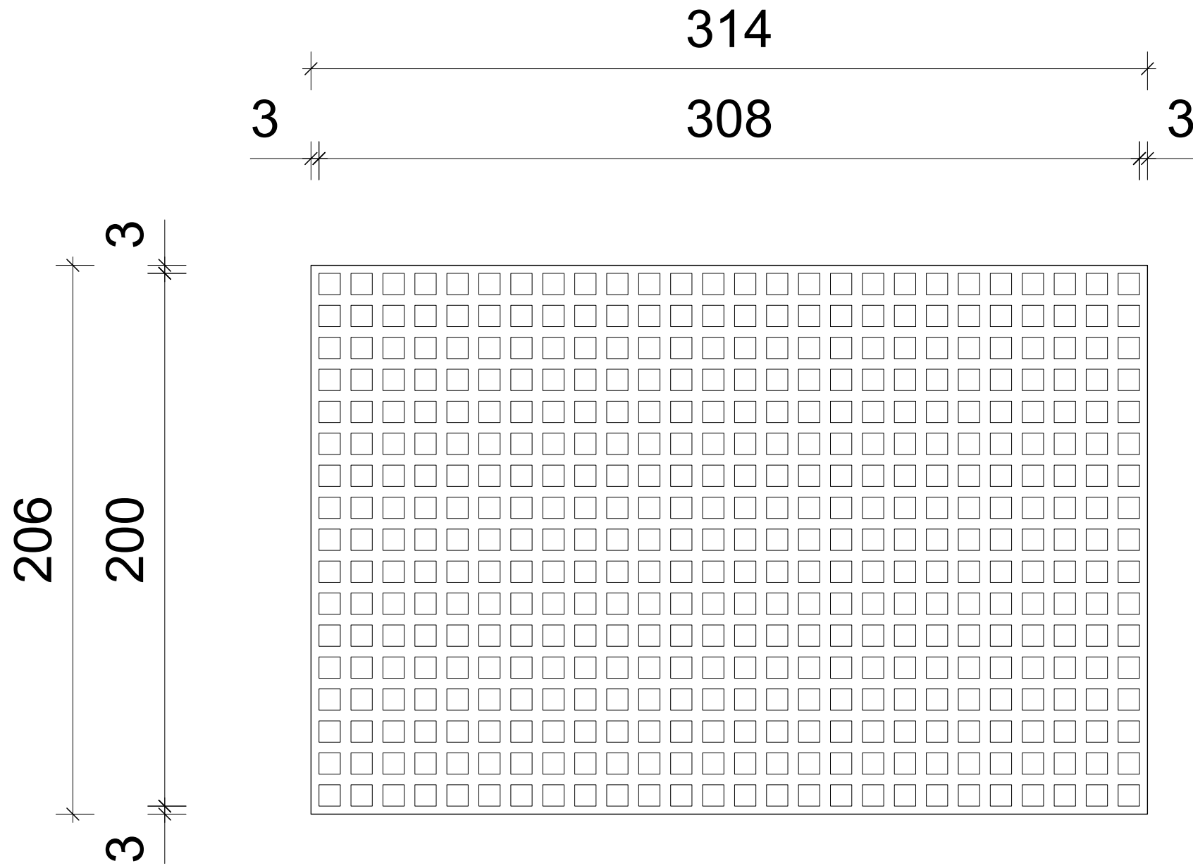
Edelstahl Lochblech 1,5mm Quadratlochung 8mm Qg 8 - 12
