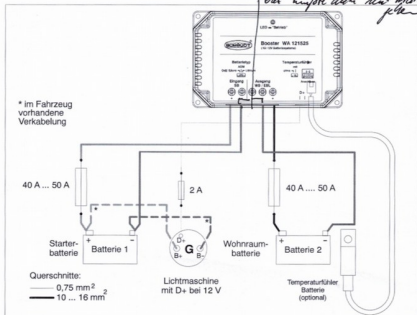
Bild 4 Fahrzeuge mit Stromversorgungen ohne Schaudt EBL ...
