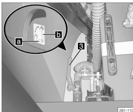
a – Ventil geschlossen b – Ventil geöffnet
