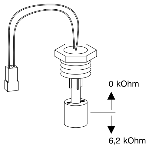
Geber Abwassertank
