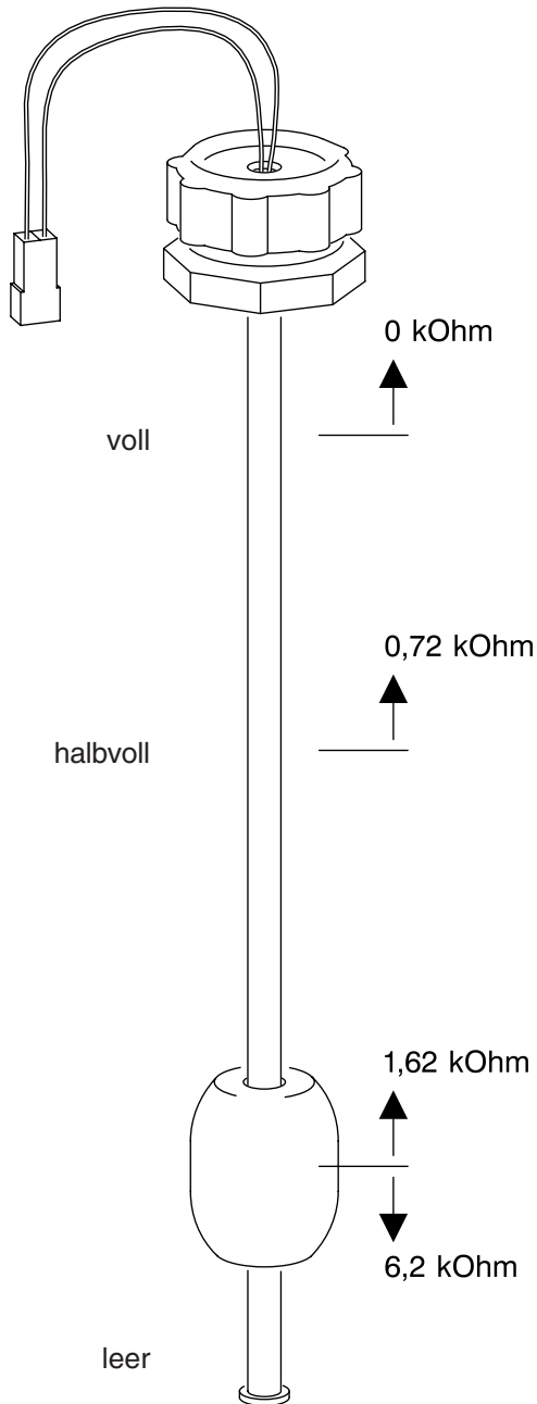
Geber Frischwassertank
